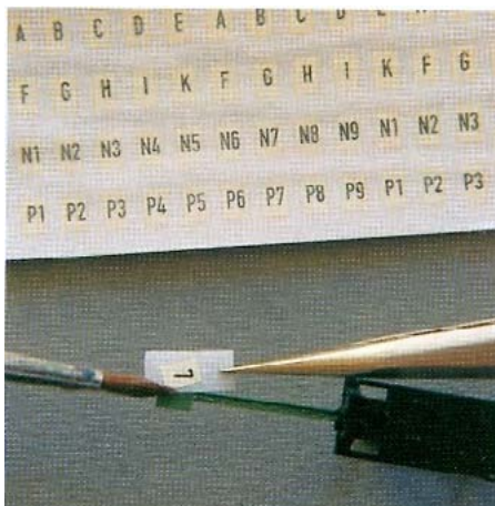
Voorbeeldgetrouw wordt het bloksein van een cijfer voorzien. Het oneven cijfer geeft al aan dat het om een sein van het spoor in telrichting gaat.
