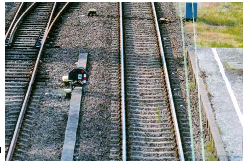
Omdat er op het linker spoor geen treinen vertrekken, is hier één spersein voldoende.
